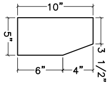
SIDE ELEV.
