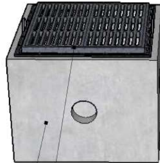
3x3 Metal Frame & Grate
