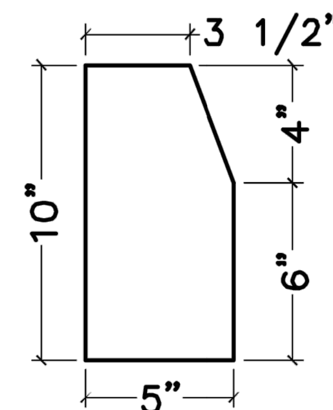
SIDE ELEV.
